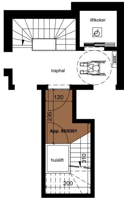
Appartement 0301 (benedenverdieping)
